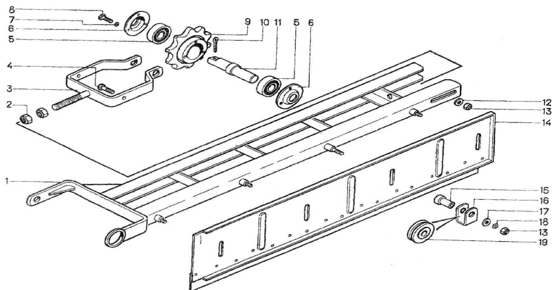
Рис. 11. Питатель ЗП 02.080
